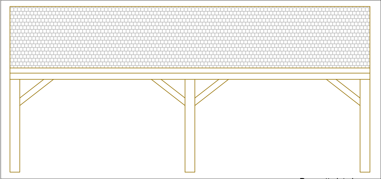
Prospetto lato lungo
